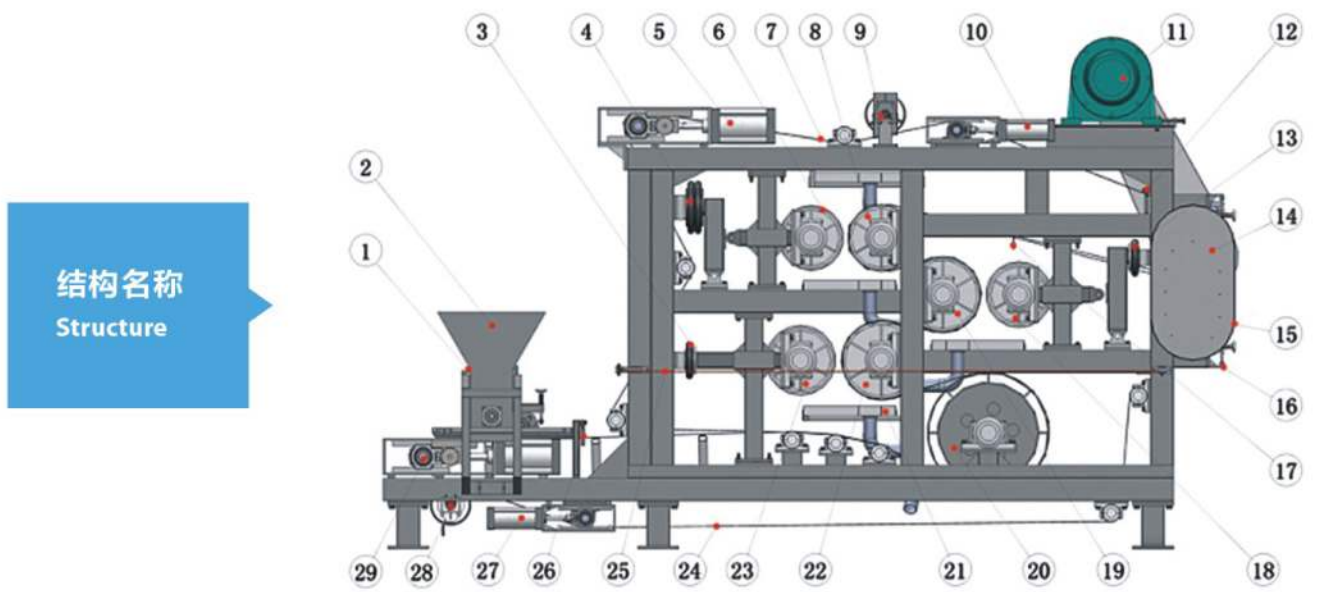
主要部件 The main components
